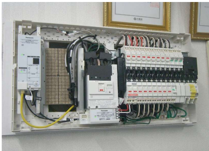
エネルギー管理システム分電盤(HEMS)
